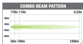
ILEDBLAST2S Op. Volt: 12-24V DC
