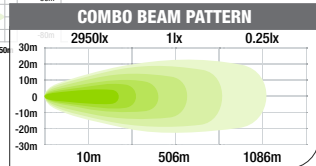
ILED9M Op. Volt: 12-24V DC
