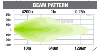
ILED7M Op. Volt: 12-24V DC
