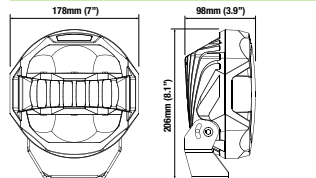
IDL0701C Op. Volt: 10-32V DC
