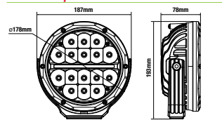
ILED7M Op. Volt: 12-24V DC
