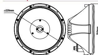
ILED9C Op. Volt: 12-24V DC
