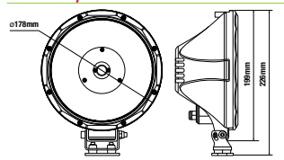
ILED7C Op. Volt: 12-24V DC
