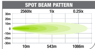
ILED7C Op. Volt: 12-24V DC
