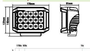
ILED5X7 Op. Volt: 12-24V DC
