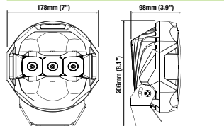
IDL0701S Op. Volt: 10-32V DC
