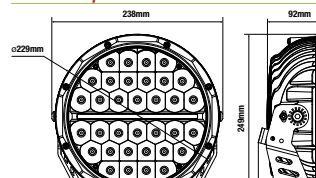
ILED9M Op. Volt: 12-24V DC
