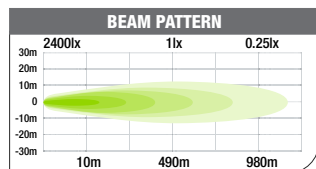
IMEGATOM Op. Volt: 9-30V DC
