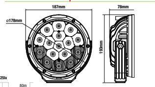
ILEDBLAST2C Op. Volt: 12-24V DC
